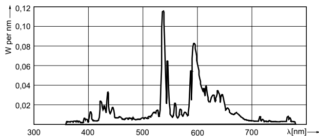
MASTERCLOUR CDM-T 20W /830
